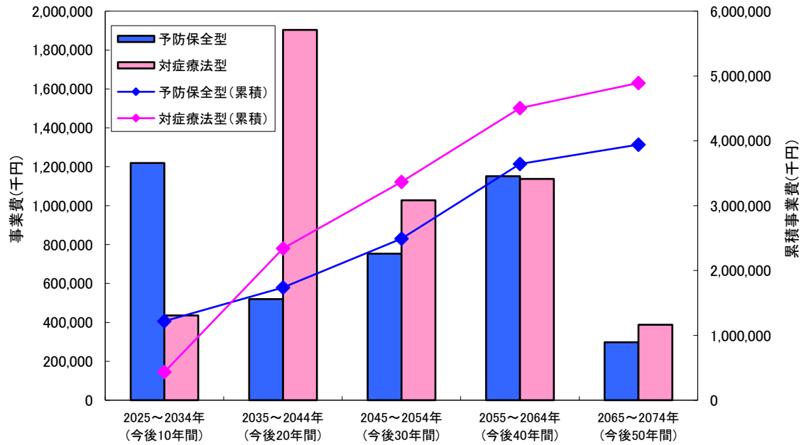
図-2 今後50年の維持管理コストの比較
